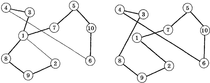
Маршрут Эйлера: 1-7-5-10-6-4-3-1-8-9-2-1
